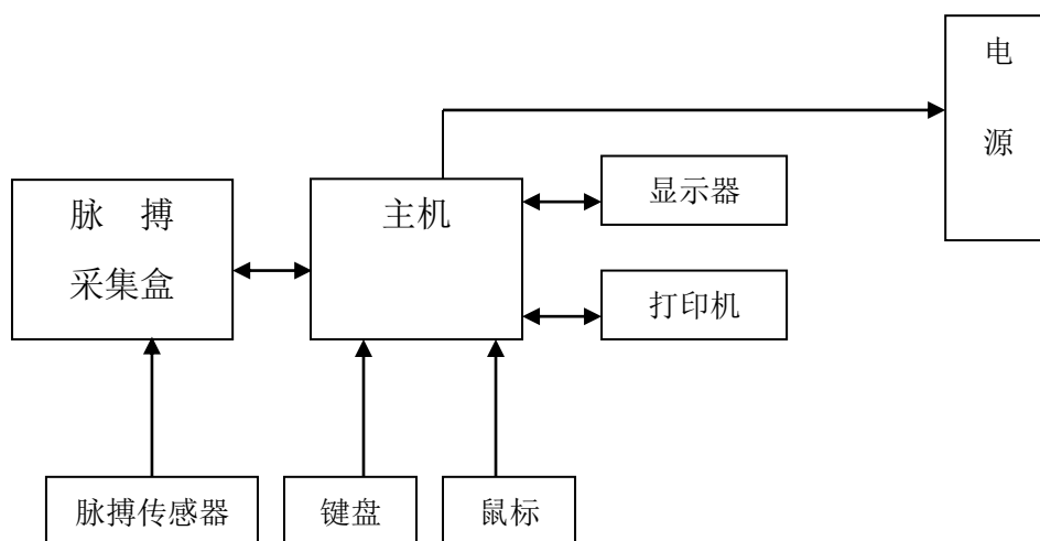
图 5-2 HK-X-A 自动心血管功能检测仪连接图
