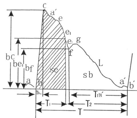
图 3.2 典型脉搏波图
