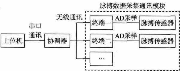
图 1 系统的拓扑结构图 Fig. 1 Topology of the whole system
