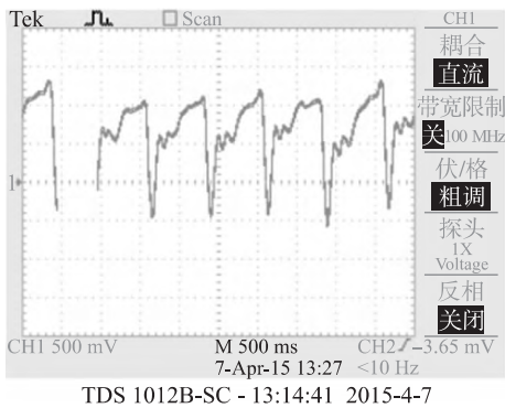
图 4 HK-2000B+脉搏传感器输出的模拟信号 Fig. 4 Pulse output signal of HK-2000B+sensor
