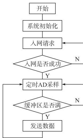
图 2 脉搏数据采集通信模块流程图 Fig. 2 The flow chart of Zigbee terminal Module
