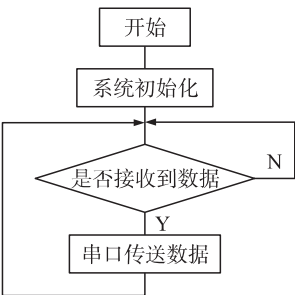
图 3 协调器软件流程图 Fig. 3 The flow chart of Zigbee coordinator Module
